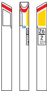
N 41: Kantpæle har gul refleks i højre og hvid refleks i venstre vejside. Kantpælens toppe hælder ned imod vejen.
